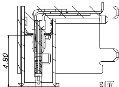
剖面 A-A
