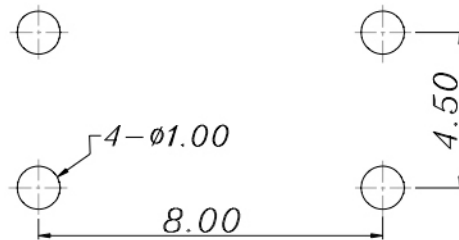
印制线路板 Recommended P.C.B layout
