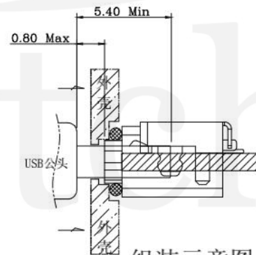
组装示意图
