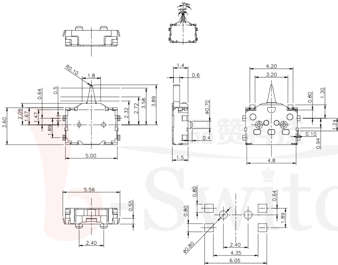
P.C.B LAND DIMENSION
