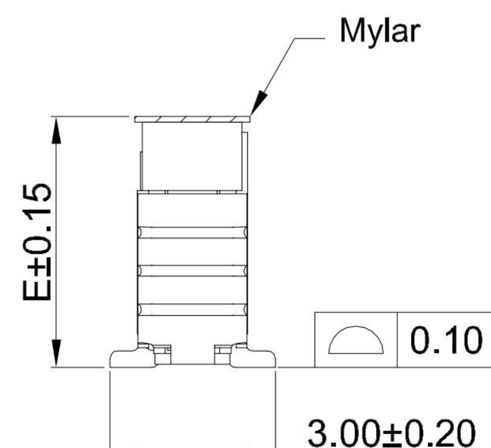
4PIN-5PIN MYLAY
