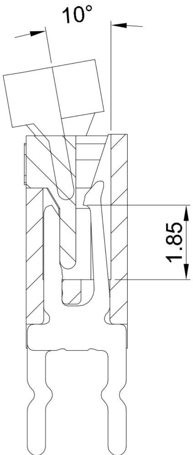
SECTION A-A
