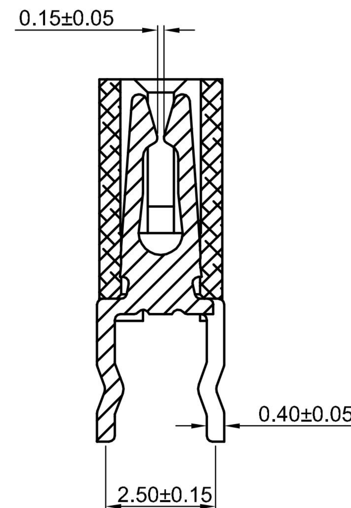
SECTION:A-A
