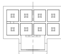
08Pin
