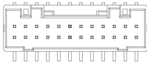
24Pin
