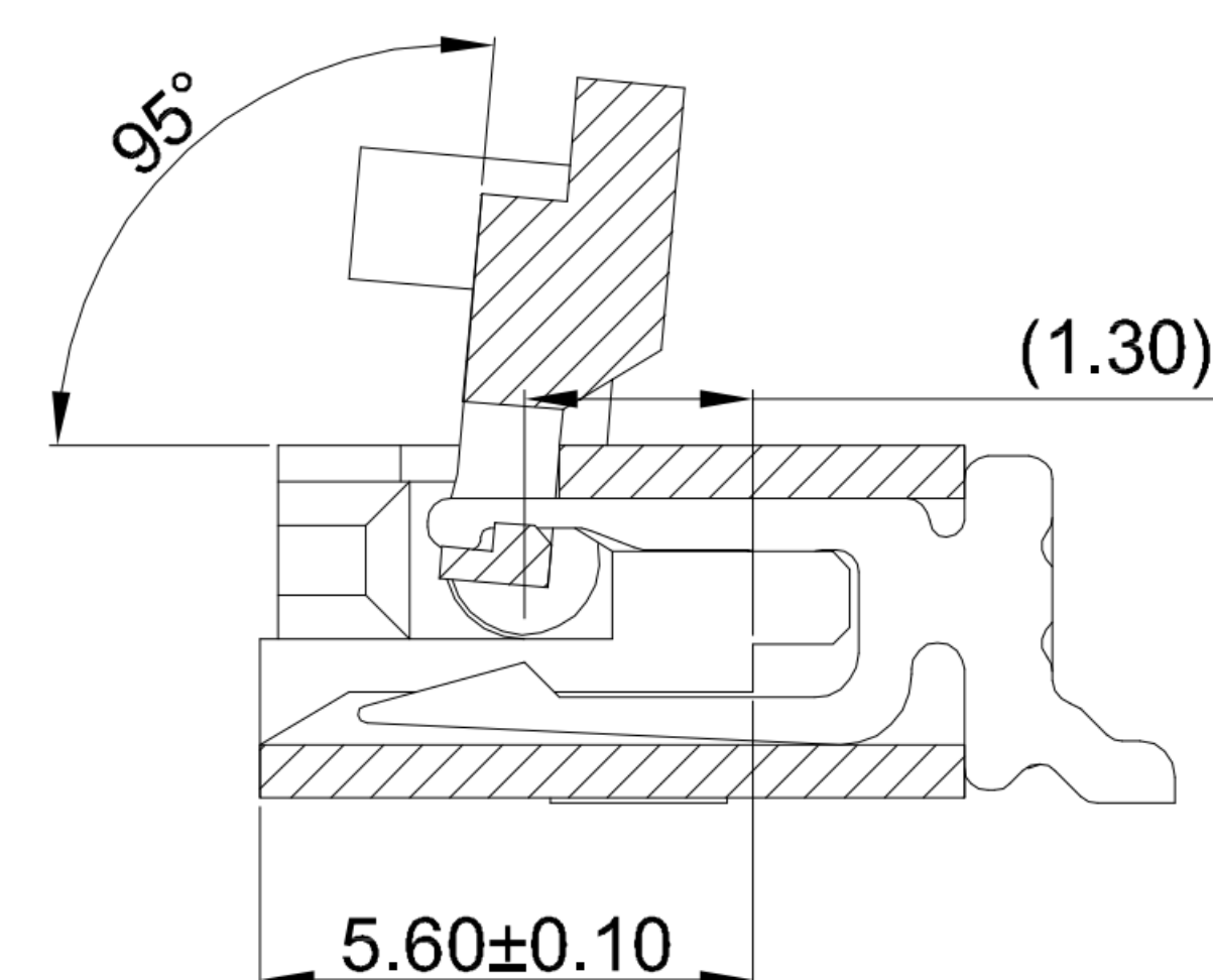
SECCION:A-A
