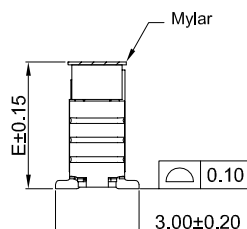
4PIN-5PIN MYLAY
