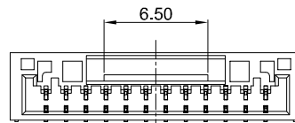
12Pin
