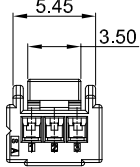
3PIN
