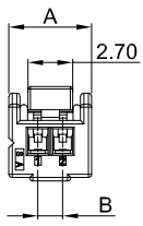
2PIN
