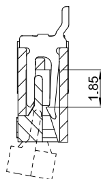
SECTION A-A
