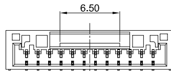
12Pin
