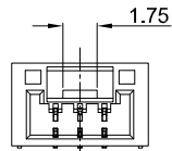
3Pin
