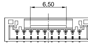
10Pin
