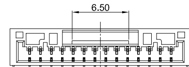
14Pin
